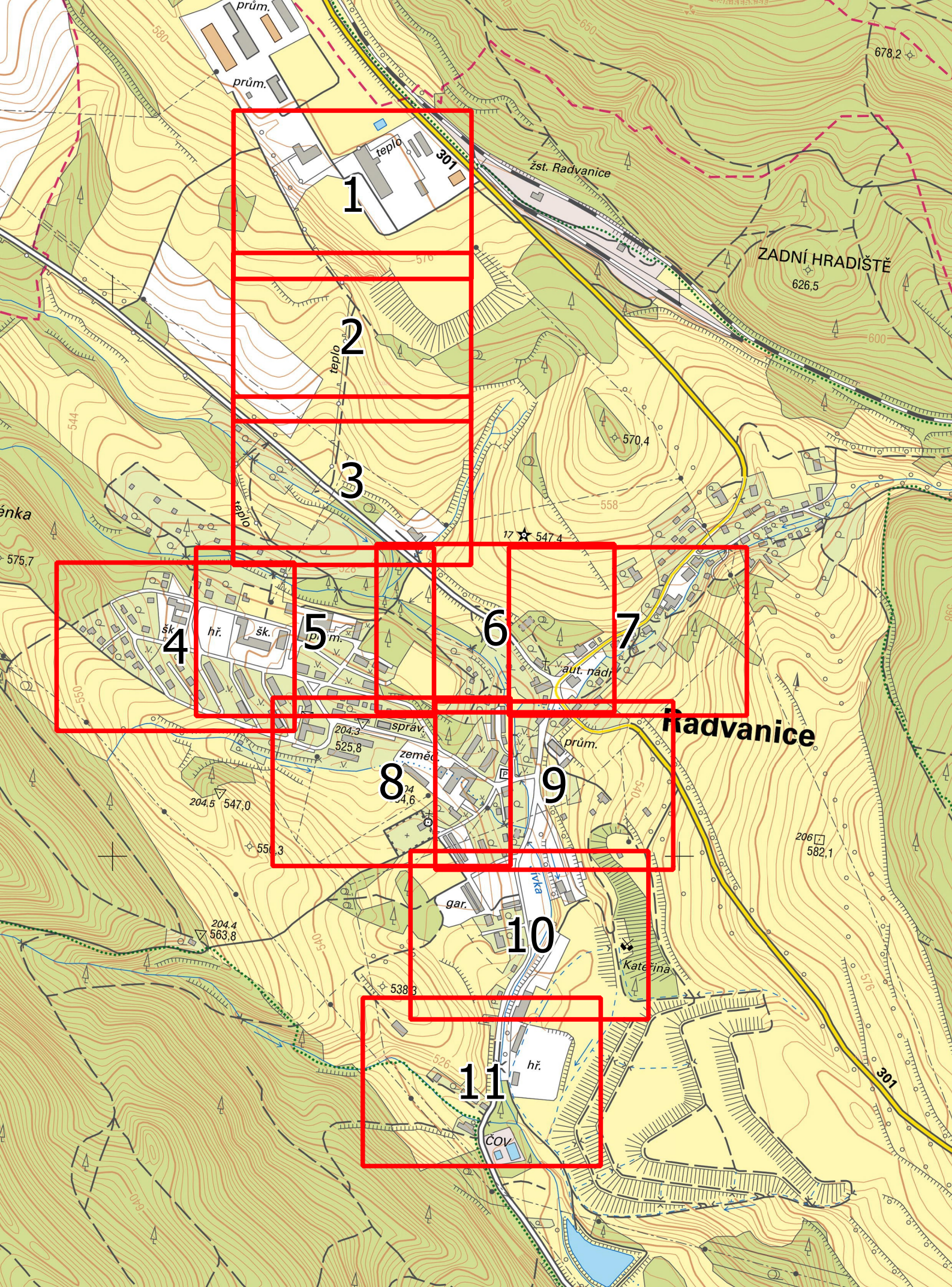
Přehledná mapa pasportu splaškové kanalizace obce Radvanice
